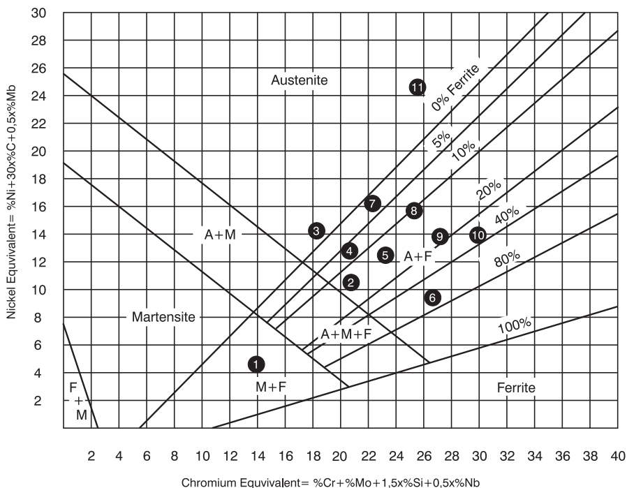
Rys. 1 - Wykres Schaeffler'a
