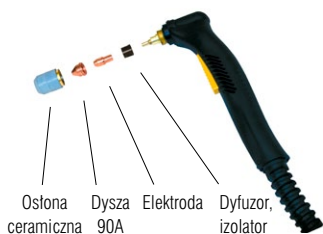
Palnik PT-38
