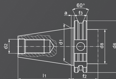
Odmiana A: bez otworu przelotowego Odmiana AD: z otworem przelotowym do centralnego doprowadzenia chłodziwa Odmiana B: do boczego doprowadzenia chłodziwa
