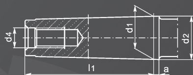
MK 2 - MK 6 Uchwyt stożkowy, z wewnętrznym gwintem dociągającym
