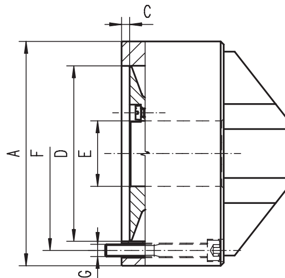
Wielkość uchwytu 85 and 110 mm
