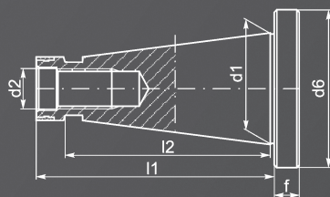
SK 30 and SK 50 Z wewnętrznym gwintem dociągającym
