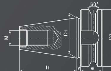
Sworznie dociągające MAS 403-BT Typ A or B
