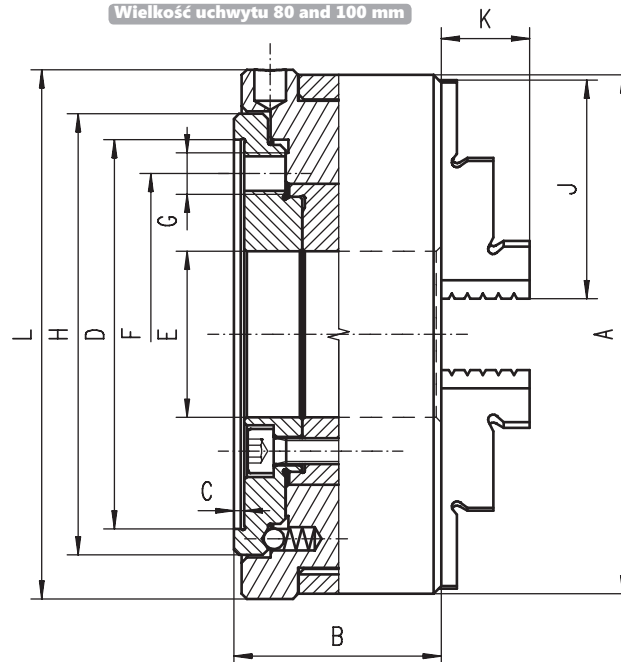
Wielkość uchwytu 80 and 100 mm
