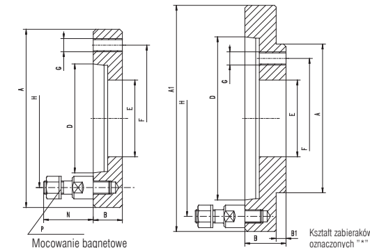
TARCZE ZABIERAKOWE OBROBIONE DO 4306, 4307
