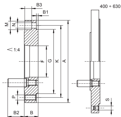
TARCZE ZABIERAKOWE OBROBIONE
