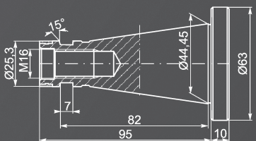
SK 40 Z wewnętrznym gwintem dociągającym, do mocowania ręcznego i z rowkiem pierścieniowym do mocowania automatycznego
