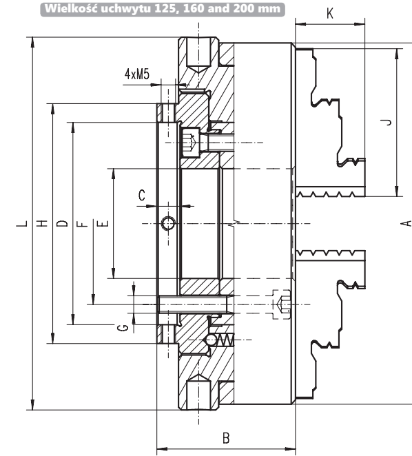
Wielkość uchwytu 125, 160 and 200 mm
