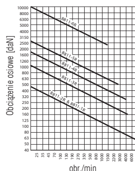
Obciążenie osiowe Trwałość łożysk - 2000 h
