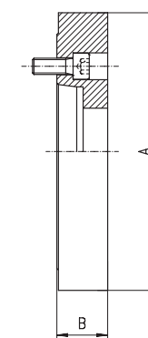
TARCZE ZABIERAKOWE NIEOBROBIONE
