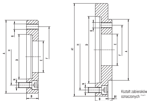
TARCZE ZABIERAKOWE OBROBIONE DO 4306, 4307
